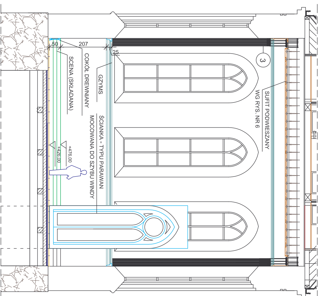
PRZEKRÓJ C-C
