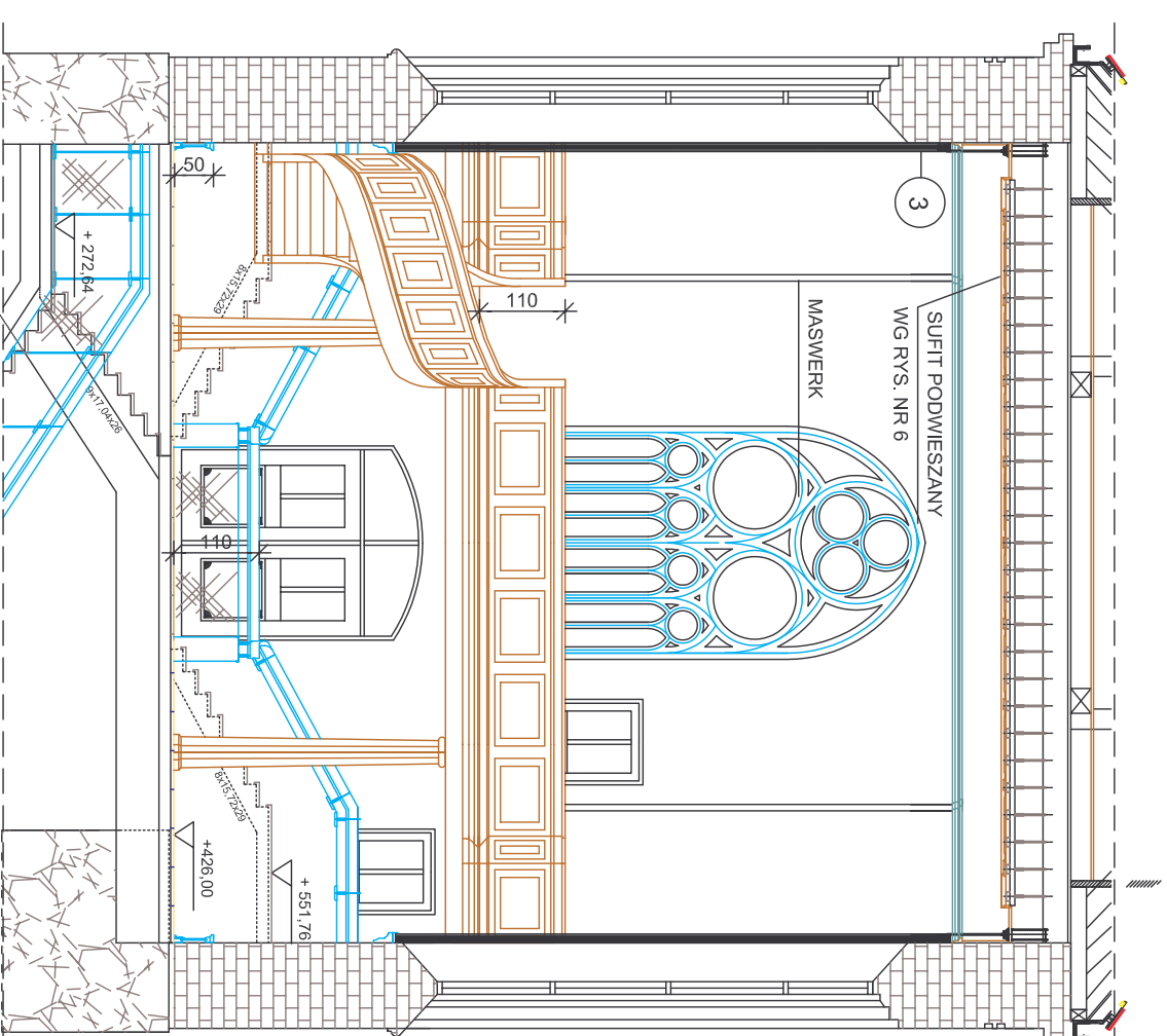
PRZEKRÓJ B-B
