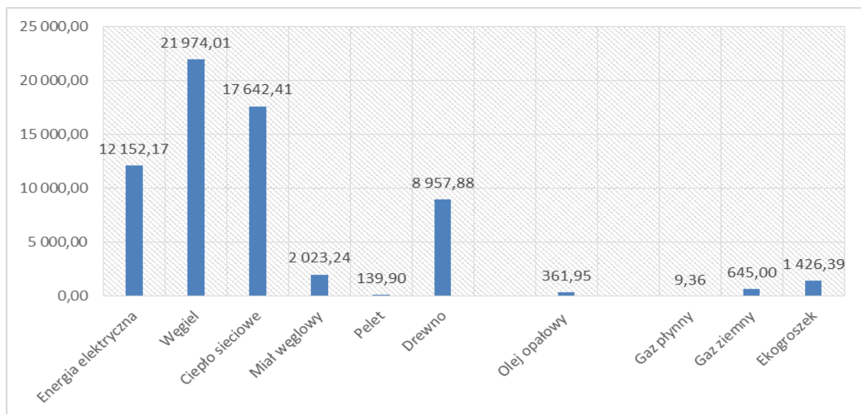
Wykres 24. Zużycie energii elektrycznej oraz paliw pierwotnych i nośników energii w 2014 r. [MWh]
