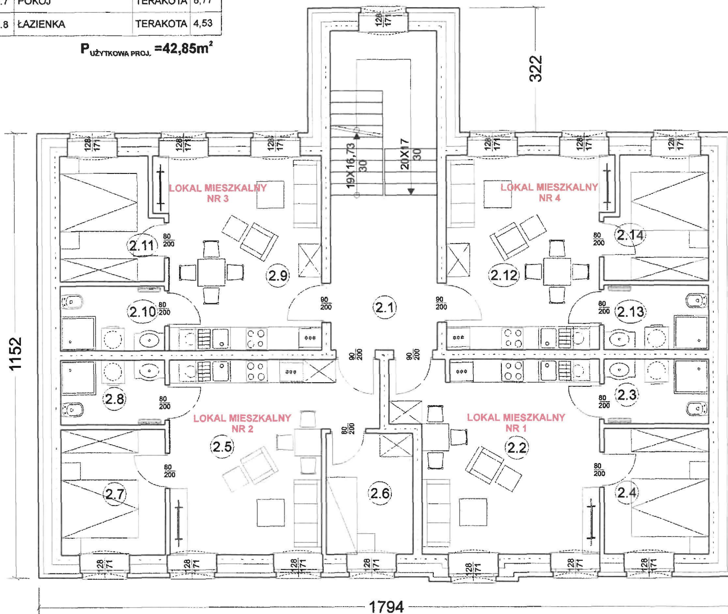
RZUT I PIĘTRA - KONCEPCJA PRZEBUDOWY, ROZBUDOWY I NADBUDOWY
