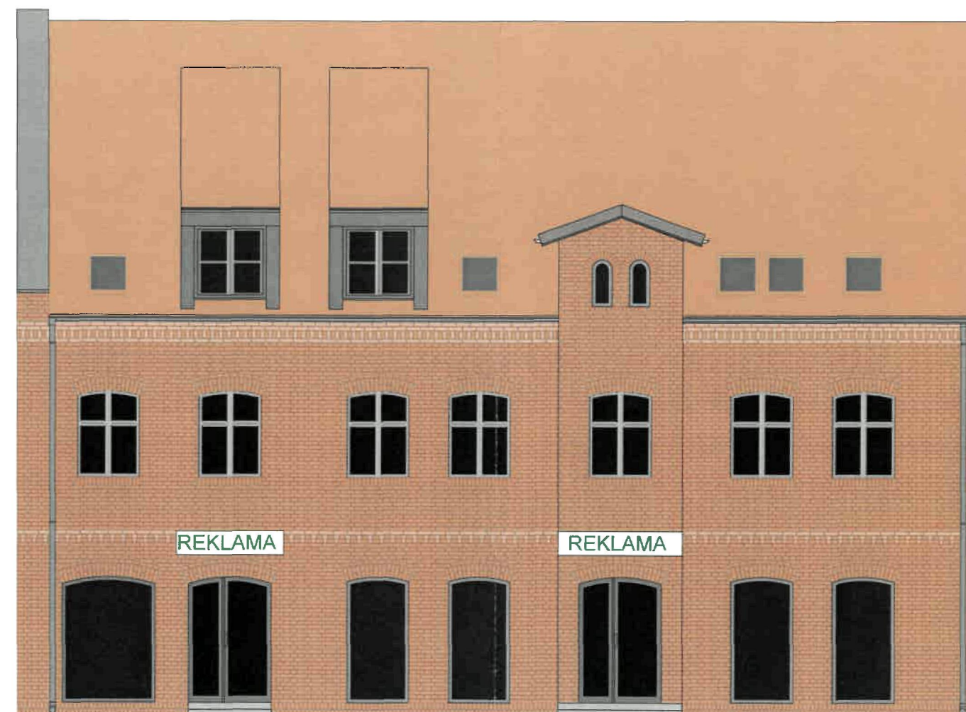
ELEWACJA FRONTOWA - KONCEPCJA PRZEBUDOWY, ROZBUDOWY I NADBUDOWY z wykorzystaniem otworów parteru witryny sklepowe
