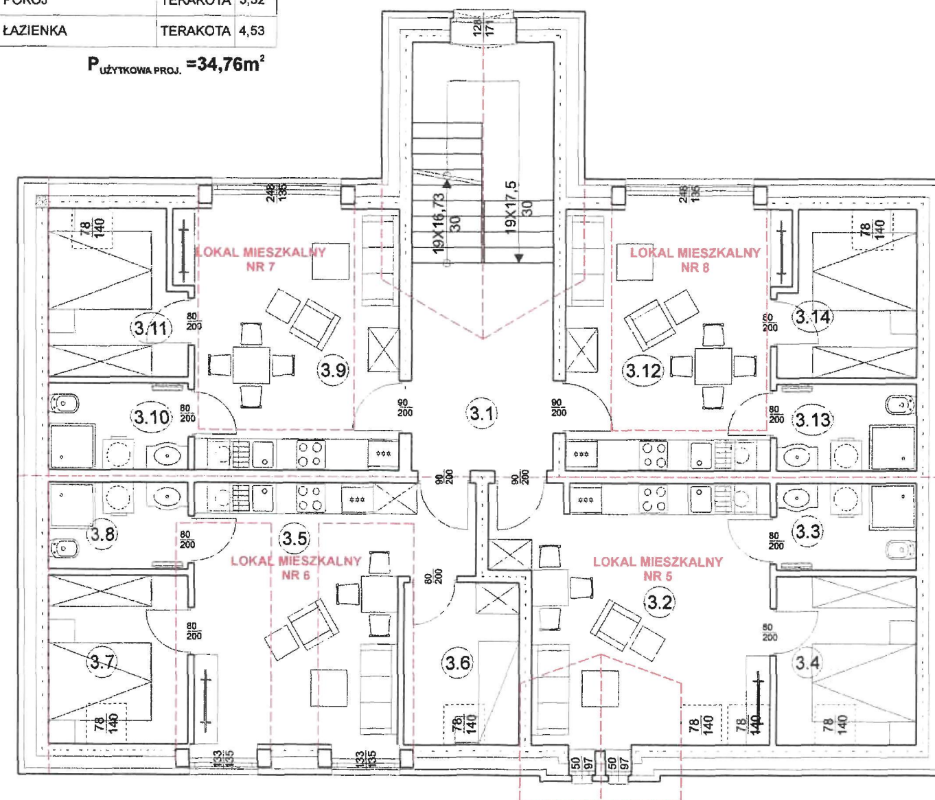
RZUT PODDASZA - KONCEPCJA PRZEBUDOWY, ROZBUDOWY I NADBUDOWY
